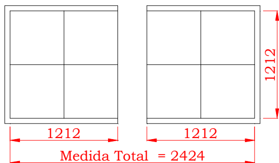
CX-4x2-2434x1212
